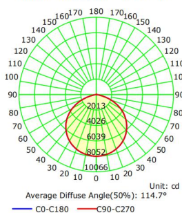
HBU2-150W
